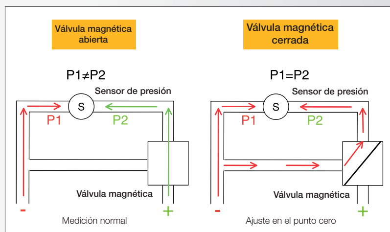
Principio de funcionamiento del ajuste automático en el punto cero de los transmisores de presión diferencial Testo
