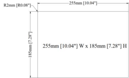
Cutout Dimensions
