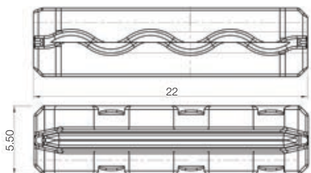
Adaptador para montaje del RTW/RPW/RNW en la lateral de contactores CWM - MARC
