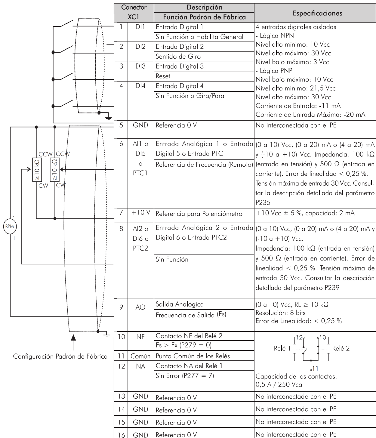
Figura 2.5 - Descripción del conector XC1 de la tarjeta de control A1 (CFW-08 Plus), tarjeta de control A2 (CFW-08 Plus con AIs (-10 V hasta +10 V)), tarjeta de control A3 (CFW-08 Plus con protocolo CANopen) y tarjeta de control A4 (CFW-08 Plus con protocolo DeviceNet)
