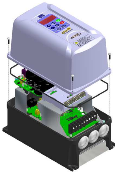
Figura 2.6 a) Posicionamiento del cierre
