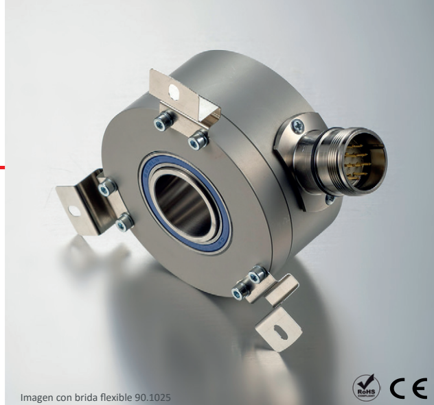
Imagen con brida flexible 90.1025
