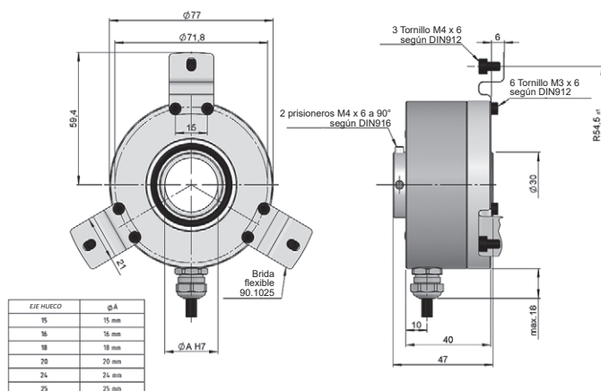
Dibujo eje hueco tipo 25, opción mecánica tipo 1 con sistema anti giro mediante brida flexible 90.1025, conexión tipo 1
