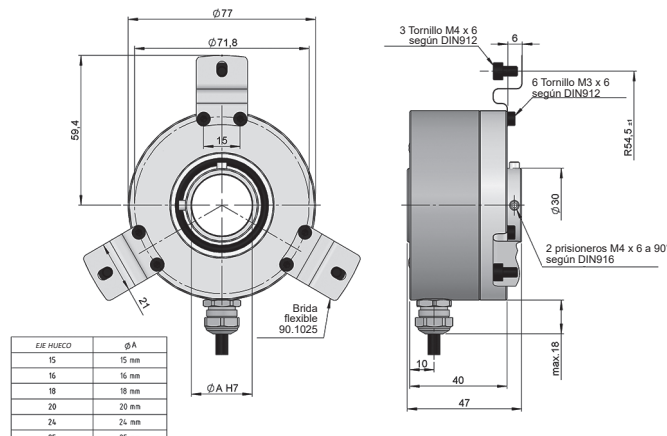
Dibujo eje hueco tipo 25, opción mecánica tipo 2 con sistema anti giro mediante brida flexible 90.1025, conexión tipo 1
