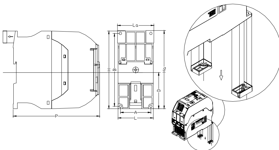
Figura 10.1 - Dimensiones de la SSW-05 Plus
