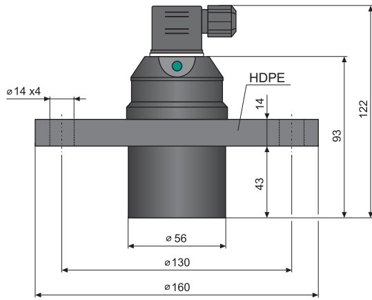
ULM-53N-10-_
