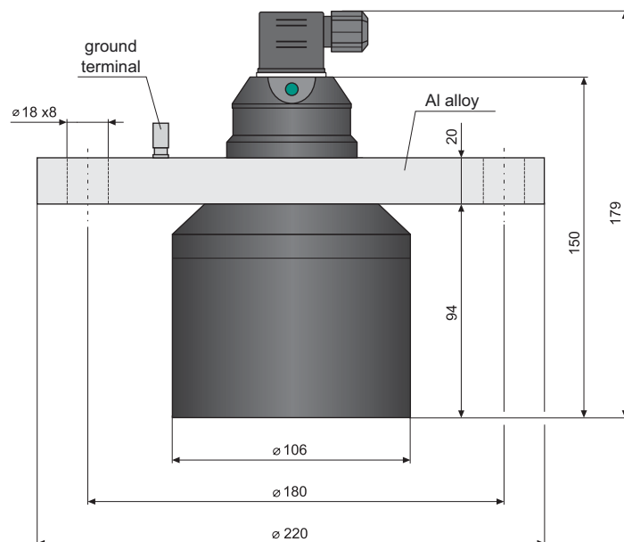
ULM-53_-20-_
