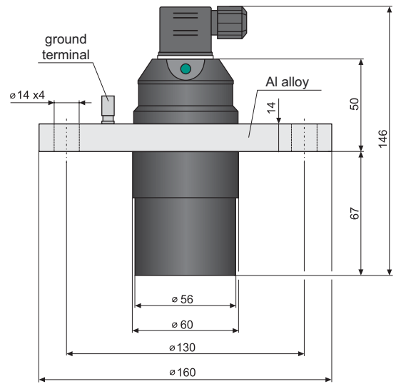
ULM-53Xi-10-I
