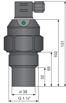
ULM-53_-06-_
