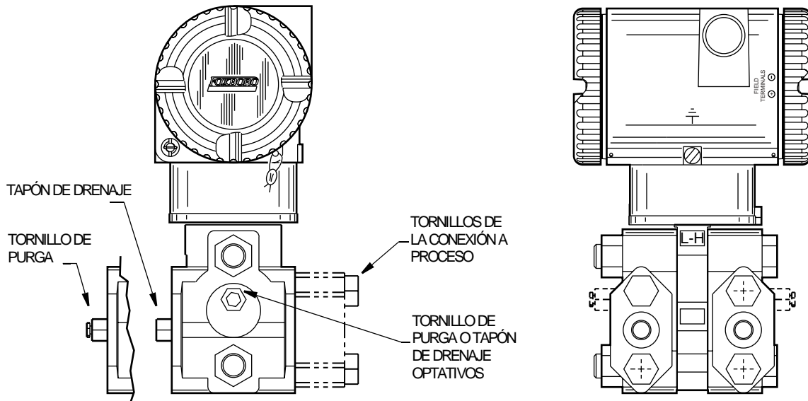
Figura 3. Conexiones de presión
